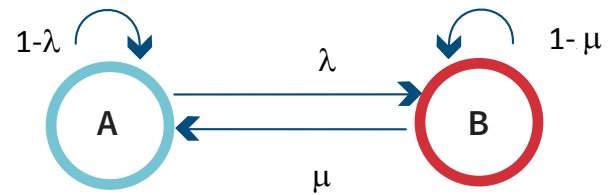
Figure 2 : Simple diagramme de transition d'états de la chaîne de Markov
